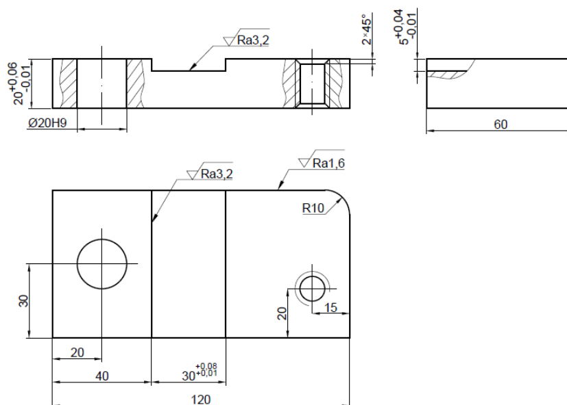
Рис. Эскиз детали (файл СМР_Зр Деталь)
