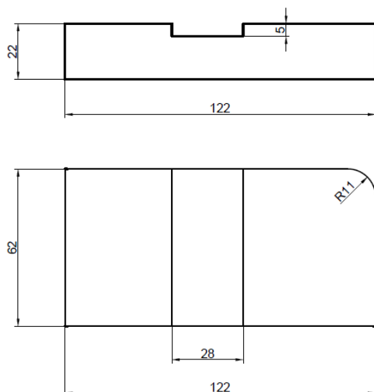
Рис. 2. Эскиз заготовки (файл СМР_Зр Заготовка)
